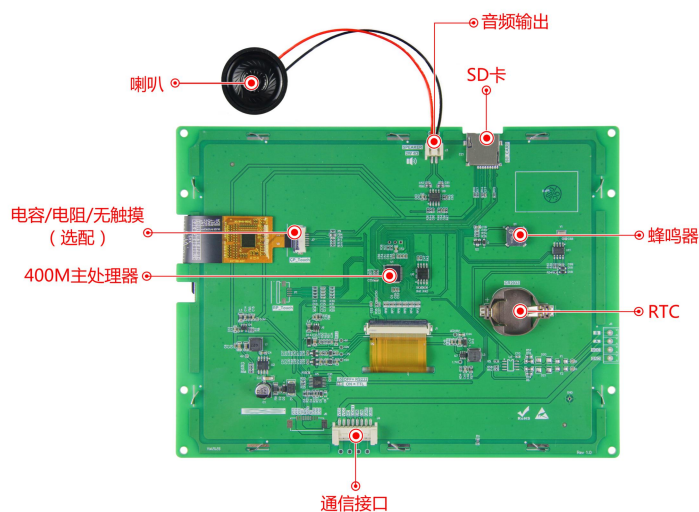
图 1-4 硬件配置图
