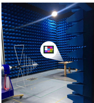
图 4-5 RE 测试图
